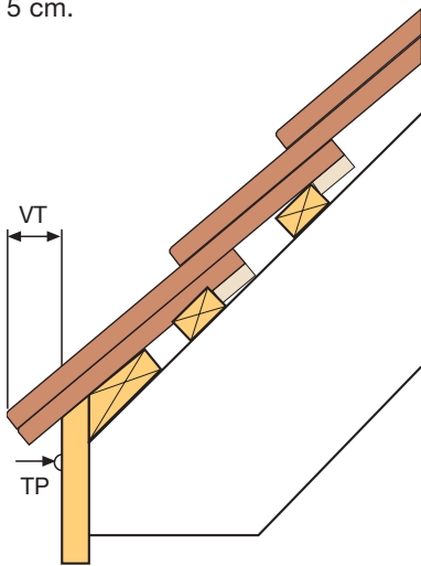
Ausgleich mit 1\frac{1}{2} -Ziegeln
