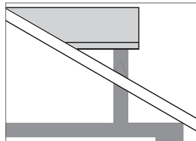
Lukarne, gegenüber der Fassade zurückgesetzt
