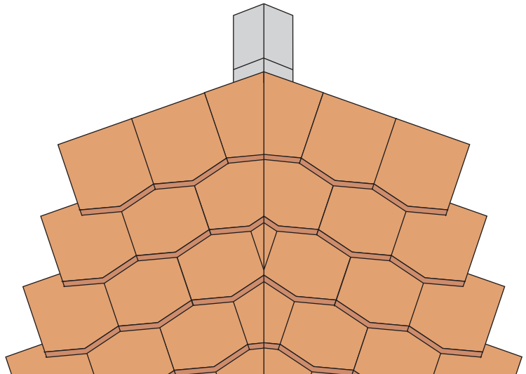
Ziegelkehle
