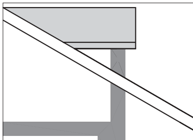
Lukarne, bündig mit der Fassade des Gebäudes
