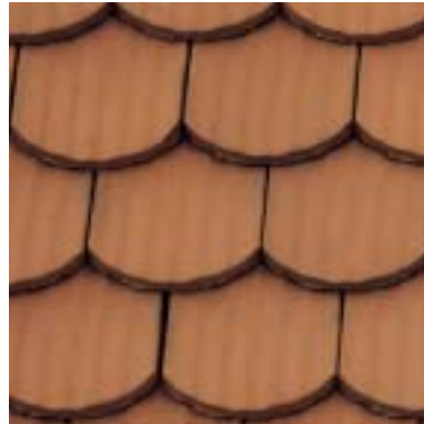
Grossflächen-Biberschwanzziegel Lattweite: ca. 20 cm Deckbreite: ca. 25 – 26 cm Ziegelbedarf: ca. 20 Stk./m 2
