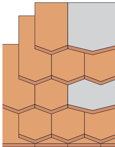
Ausgleich mit 1\frac{1}{2} -Ziegeln
